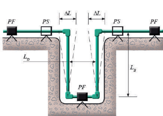
Ejemplo de brazo de compensación en forma de "Ω" Example of "Ω-shaped" compensation arm.
